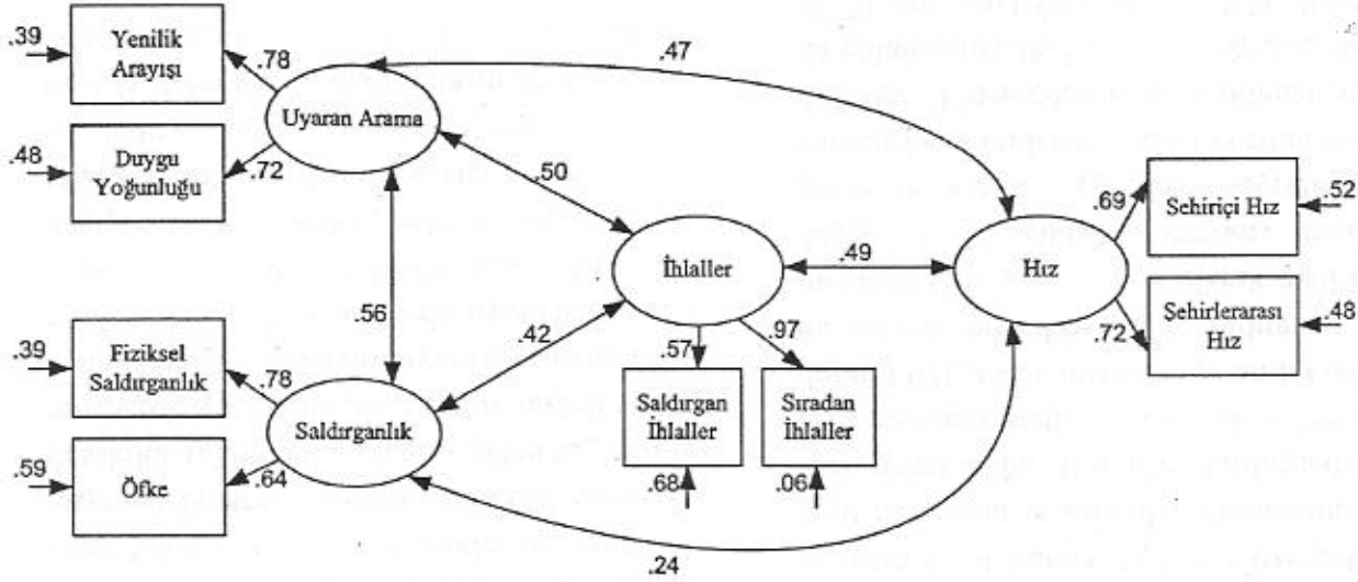
Şekil 4. Örnek Uygulama: Doğrulayıcı Faktör Analizi
