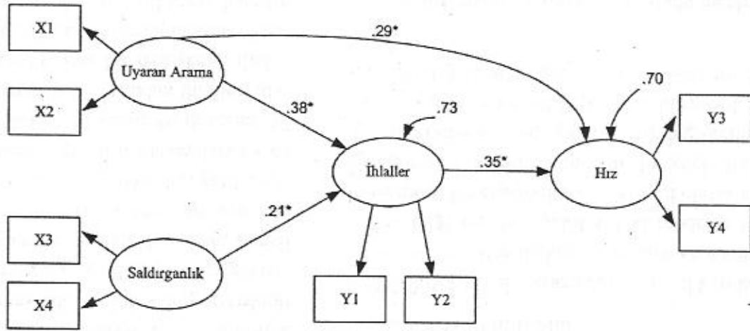
Şekil 5. Örnek Uygulama: Yapısal Eşitlik Modeli
